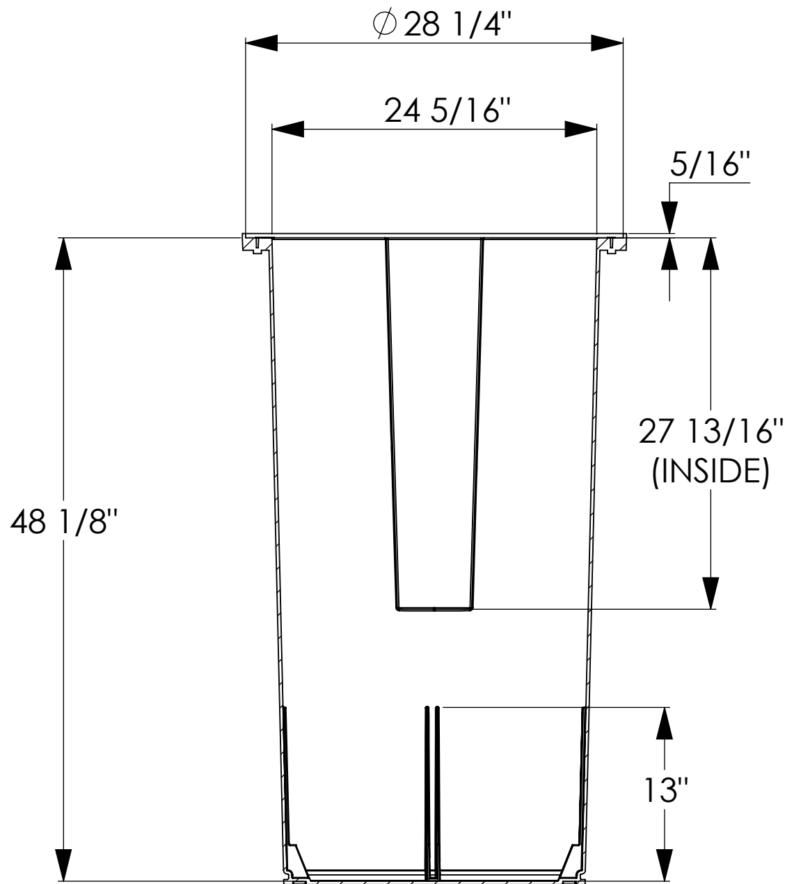
SECTION A-A
